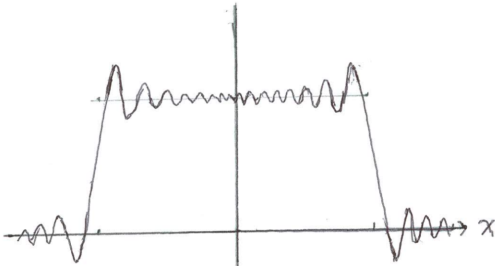
\text{Re } e^{it\Delta} \chi_I(x)
